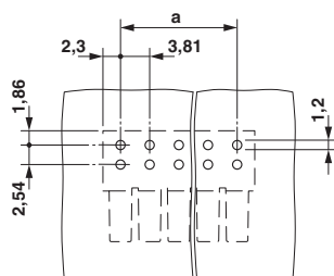
Vrtací schéma
